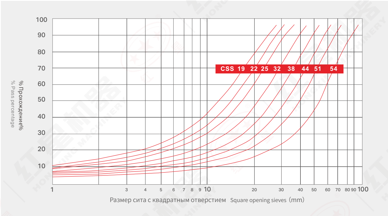
кривая распределения частиц в SC - S SC-S medium crushing Indicative gradation curve
