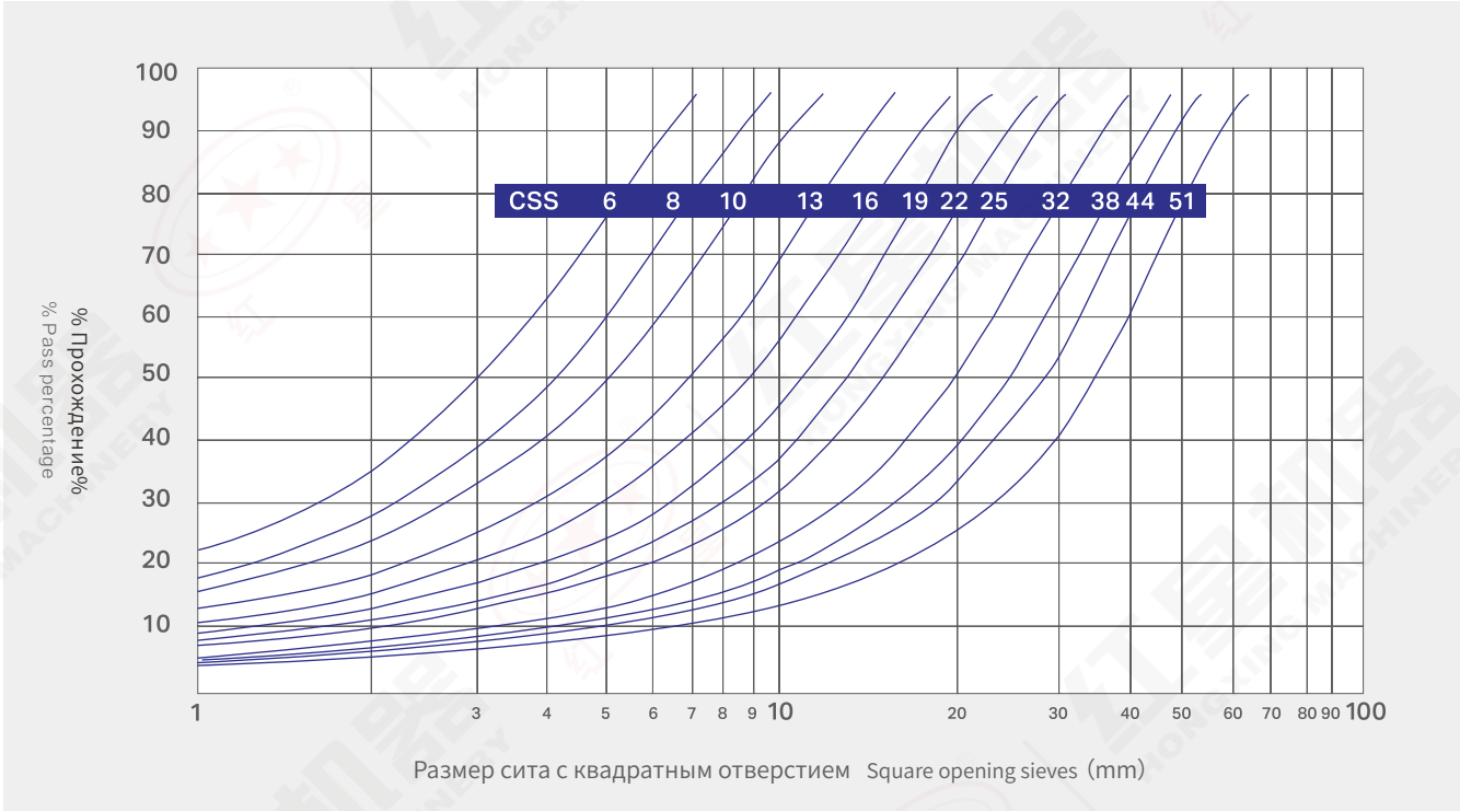
SC кривая распределения мелких частиц SC fine crushing Indicative gradation curve
