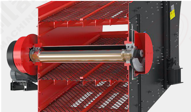
Усовершенствованная система смазки жидким маслом Advanced thin oil lubrication system
