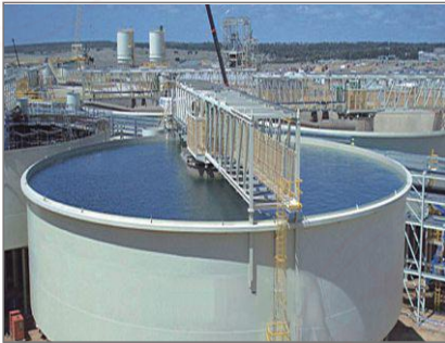
Эффективный концентратор HIGH EFFICIENCY CONCENTRATOR
