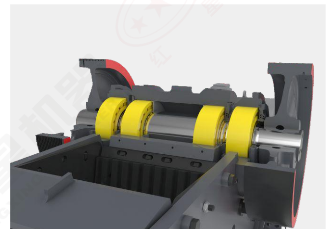
Увеличенные подшипники той же спецификации Oversized bearings of the same specification
