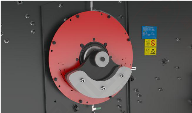
HX -- одна ось HX single axis Максимальная возбуждающая сила составляет 3,5G, что значительно повышает производительность скрининга. The maximum excitation force is 3.5G, significantly improving the screening performance.
