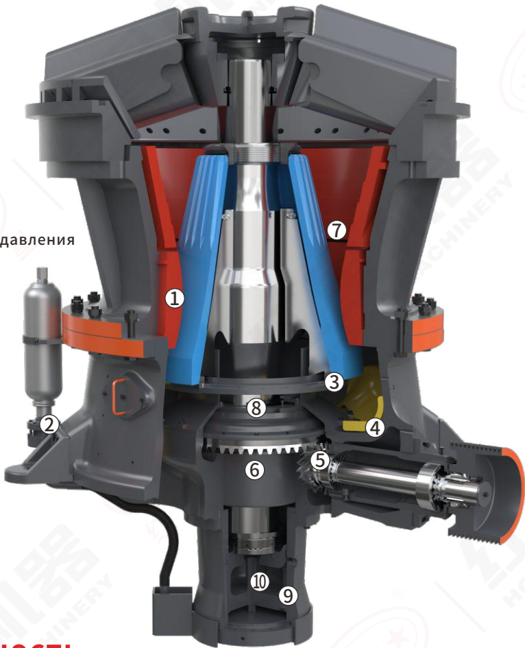
Производственная мощность конусной дробилки среднего дробления серии SC SC (S) Series Intermediate Cone Crusher Production Capacity
